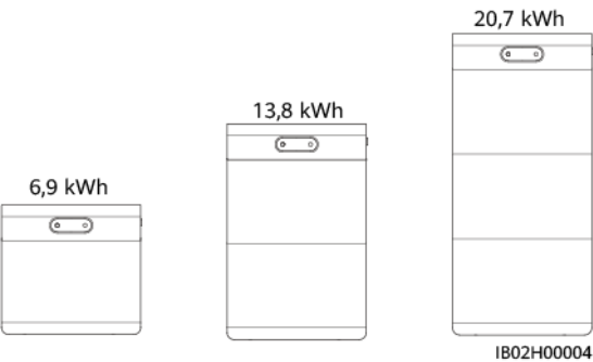
Abbildung 2-4 Kapazitätserweiterung mit Energiespeichersmodulen
