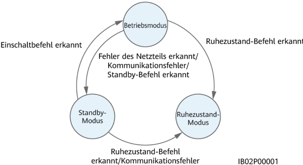
Abbildung 2-13 Umschaltung des Arbeitsmodus
