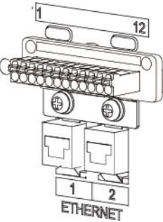
Abbildung 5-5 Signalanschluss
