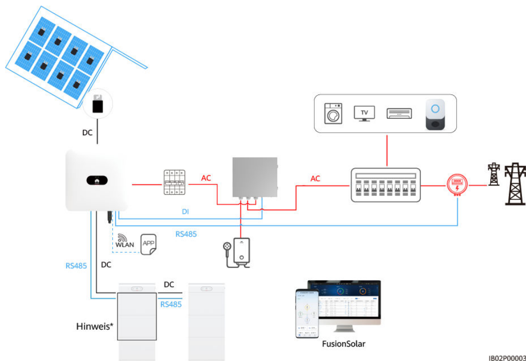
Abbildung 2-8 Netzgekoppeltes/-entkoppeltes Szenario
