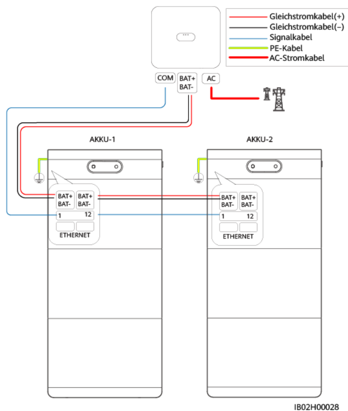
Abbildung 3-1 Kabelverbindungsplan
