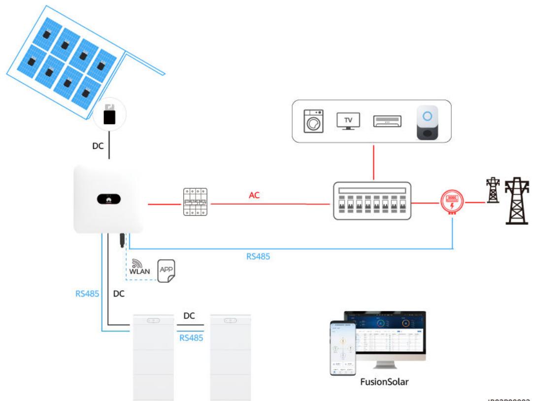
Abbildung 2-7 Netzgekoppeltes Szenario
