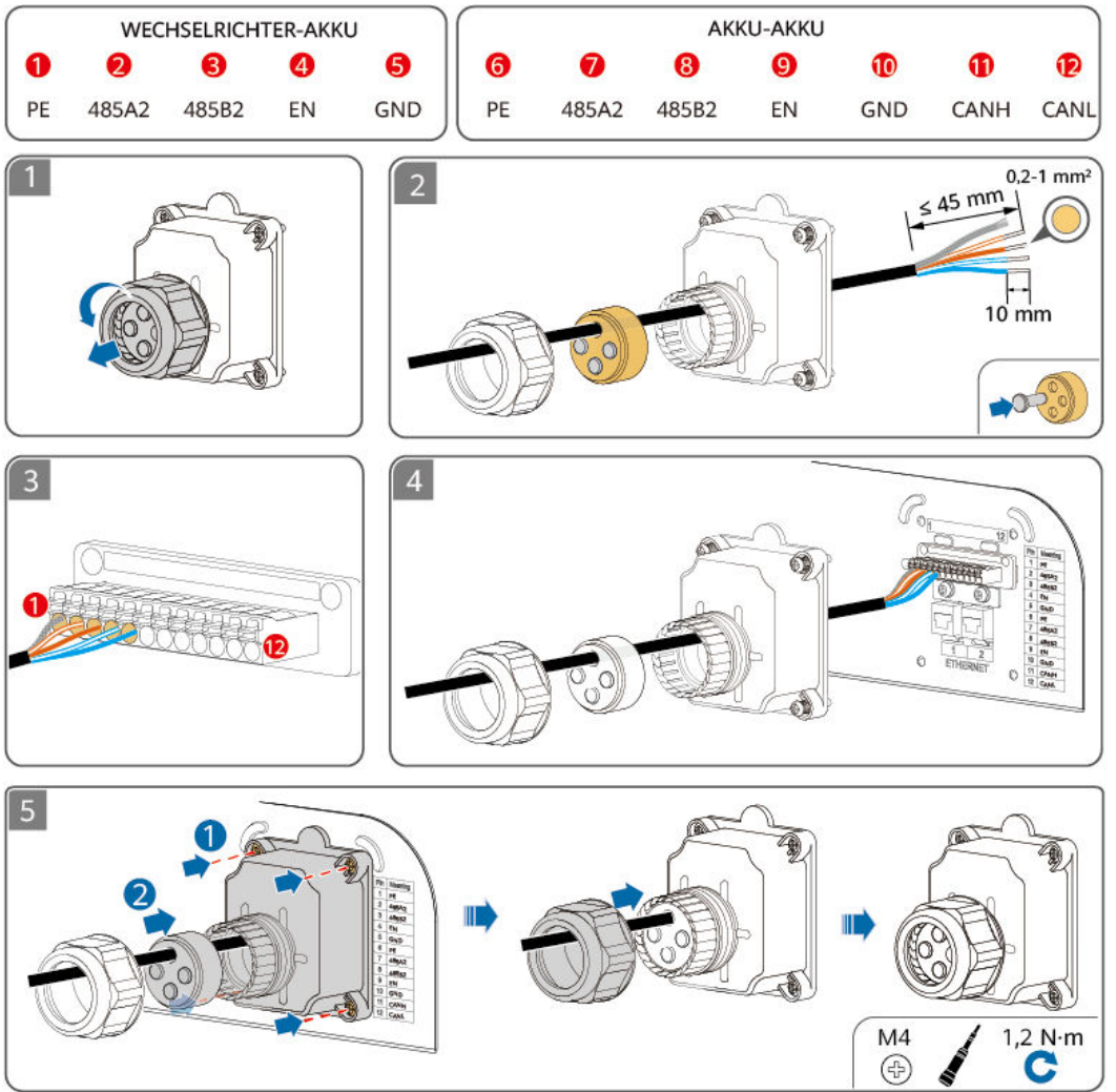
Abbildung 5-6 Signalanschlussverbindungen
