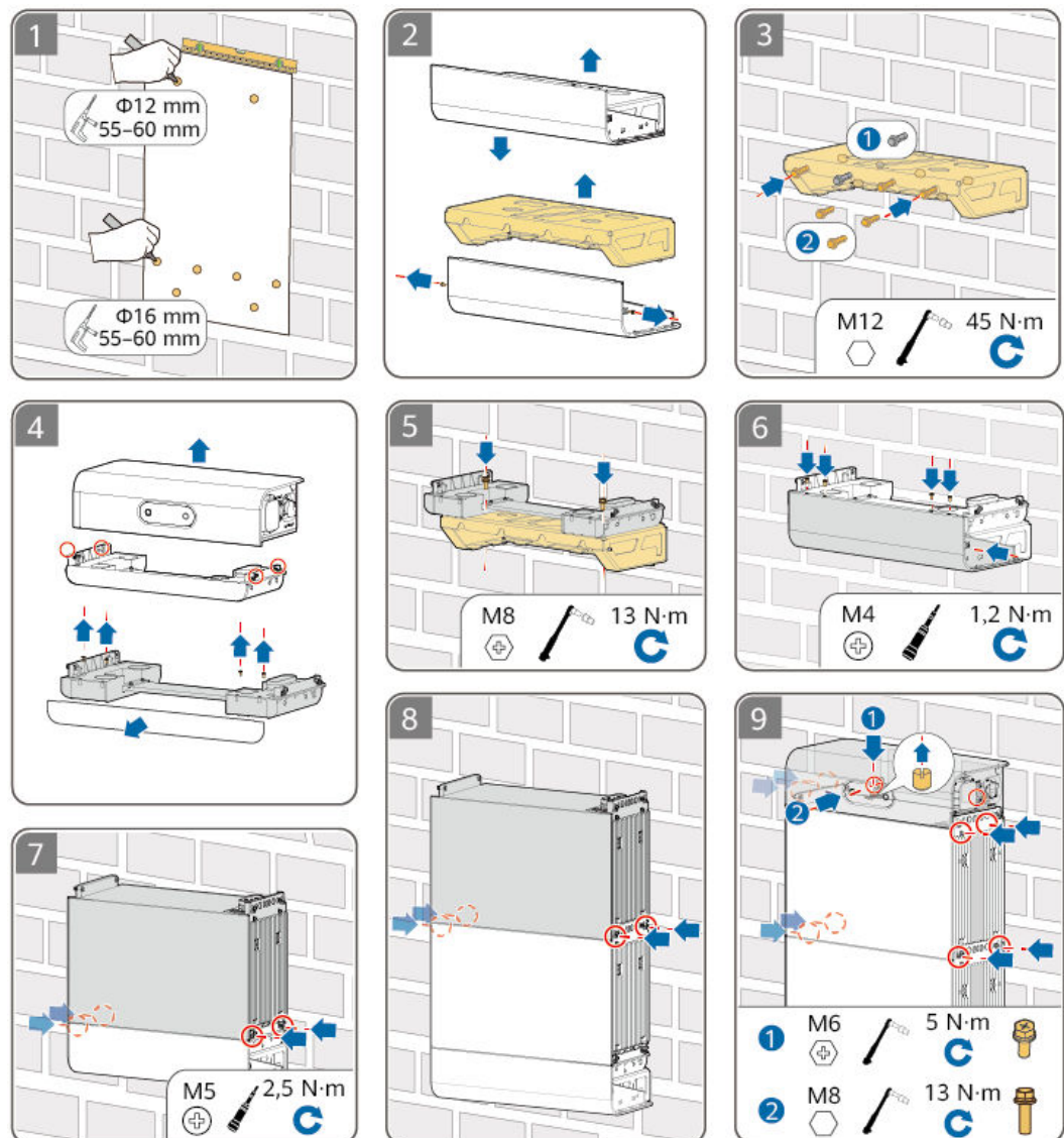
Abbildung 4-6 Wandmontage
