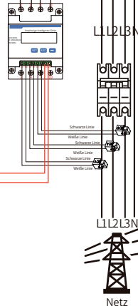
Abb. 7.14 Anschlussplan des CHINT-Zählers
