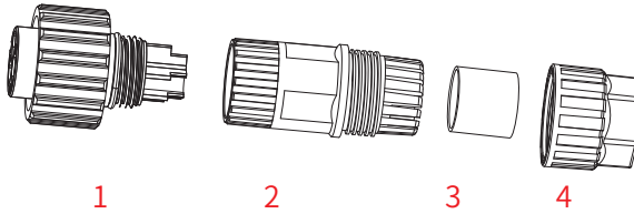
Abb. 5.7 Aufbau des AC-Steckers
