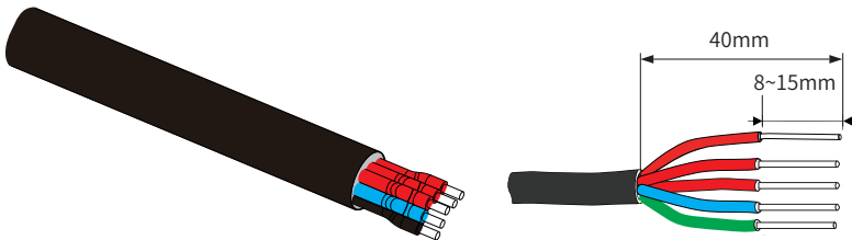
Abb. 5.8 AC-Kabel abisolieren
