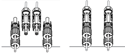
Abb. 5.6 DC-Eingangsanschluss
