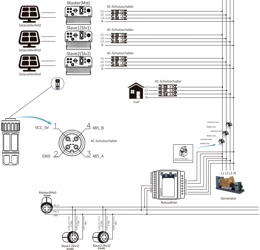
Abb. 7.25 Anschlussplan (Dreiphasenstrom)
